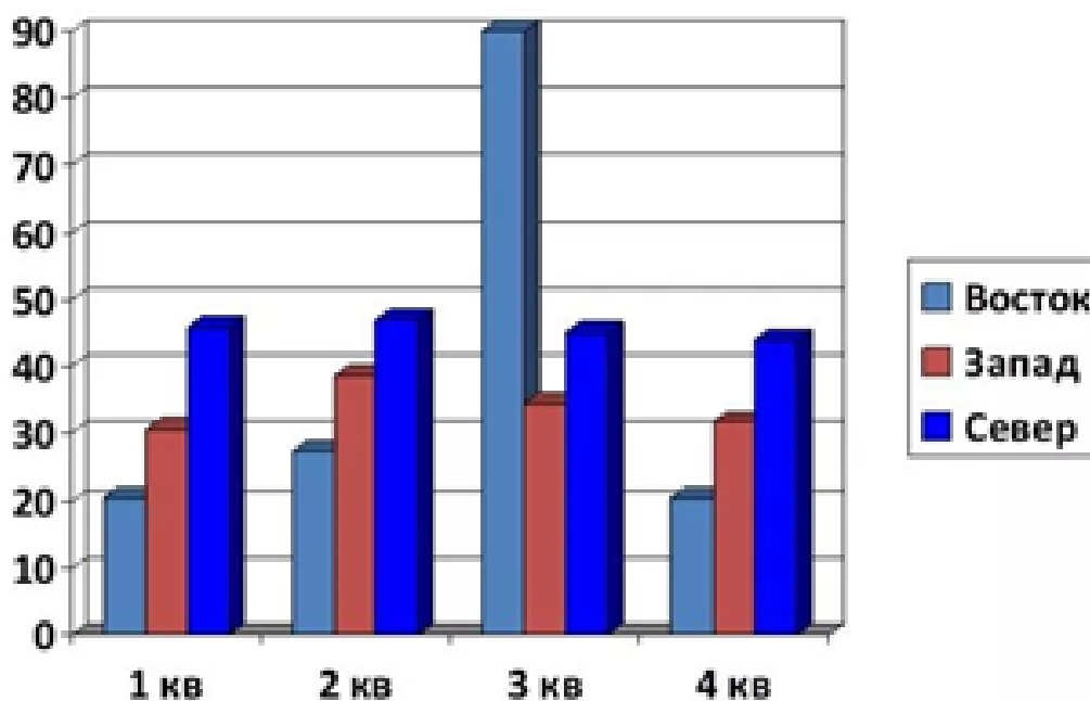
Рисунок 30. Образец гистограммы
